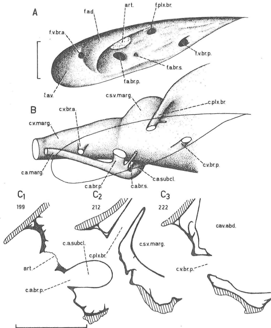
Fig. 12. — Norselaspis glacialis n.g., n.sp. A, aire d'attache de la nageoire gauche, d'après SVD 1025-1026, vue postéro-latérale ; B, canaux et cavités internes de la région scapulaire gauche, d'après les polissages sériés de SVD 1025a, vue postéro-latérale, contour de l'aire d'attache indiqué par un trait simple ; C, coupes transversales de la région scapulaire droite de SVD 1025, au niveau du foramen pour l'artère brachiale principale (C 1), de celui pour le plexus brachial (C 2) et de celui pour la veine brachiale postérieure (C 3). Echelle : 1 mm.
