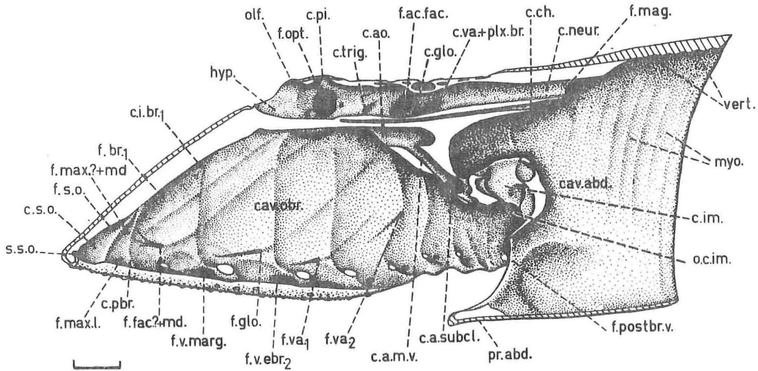
Fig. 7. — Norselaspis glacialis n.g., n.sp. Coupé sagittale du bouclier, principalement basée sur SVD 1026 et sur la série de polissages effectués sur SVD 1025. Section de l'exosquelette en hachuré et de l'endosquelette en blanc. Echelle : 1 mm.
