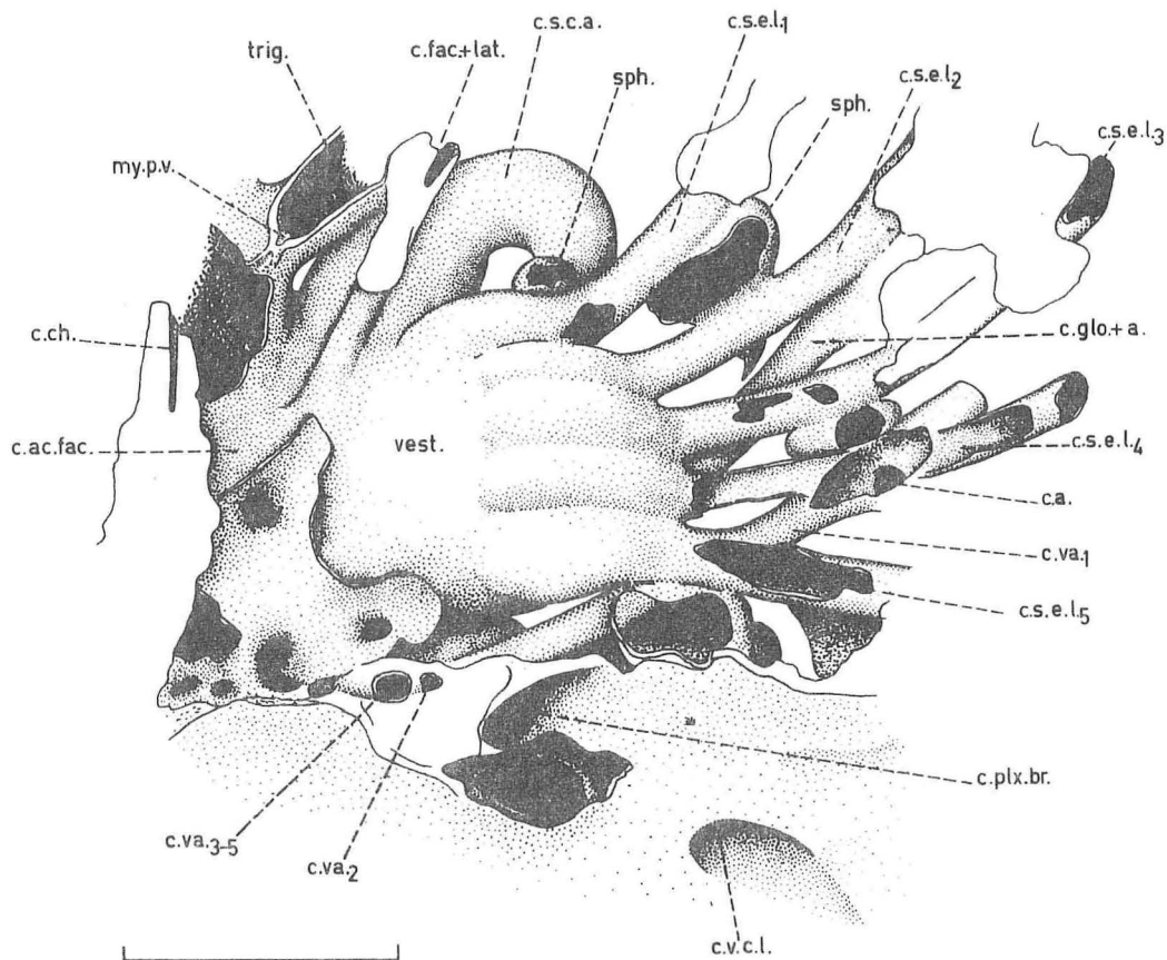
Fig. 23. — Norsespisp glacialis n.g., n.sp. Dessin à la chambre claire de la cavité labyrinthique gauche et des canaux adjacent chez SVD 1026a, préparé à l'acide formique, montrant principalement le canal pour le nerf glossopharyngien. Vue ventrale. Echelle : 1 mm.
