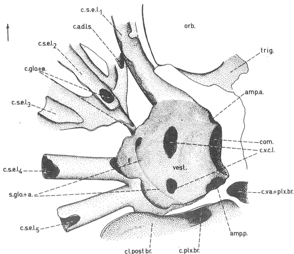
Fig. 26. — « Boreaspis puella » (WÄNGSJÖ), Formation de Wood Bay, Sigurdfjellet, Spitsberg. Dessin à la chambre claire de la paroi dorsale de la cavité labyrinthique droite et des canaux adjacents chez SVD 1018 préparé à l'acide formique, montrant notamment le sillon pour le nerf glossopharyngien et l'artère dorso-latérale superficielle. Vue ventrale. Echelle : 1 mm. La flèche indique l'avant.
