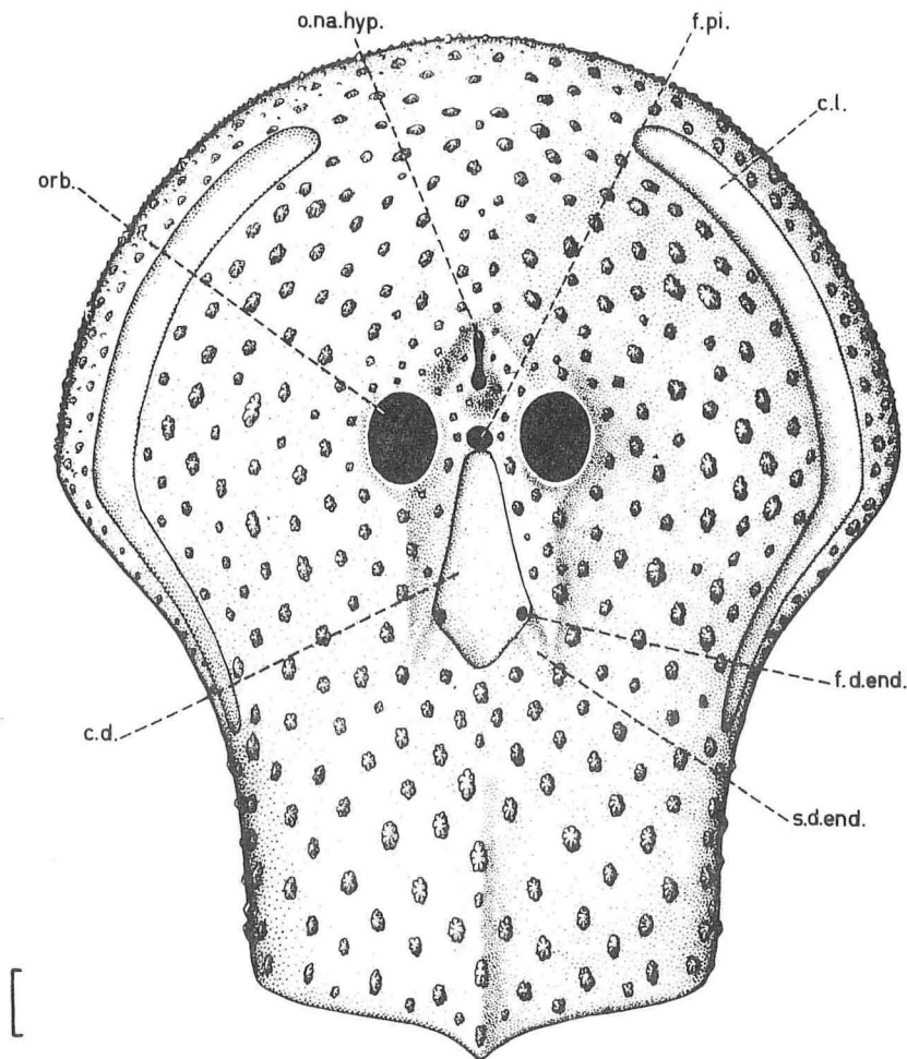
Fig. 2. — Norselaspis glacialis n.g., n.sp., Formation de Wood Bay, Division de Sigurdfjellet (Dévonien inférieur), Sigurdfjellet, Spitsberg. Reconstitution du bouclier basée sur SVD 1025 et SVD 1026 (Muséum national d'histoire naturelle, Paris), vue dorsale. Echelle : 1 mm.
