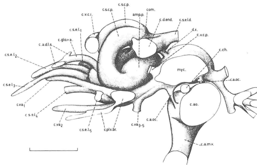
Fig. 24. — Norsespaspis glacialis n.g., n.sp. Moulage interne des canaux et cavités de la région otico-occipitale. Vue postérieure, montrant le complexe des canaux pour les branches du nerf vague. Reconstitution graphique basée sur les polissages sériés de SVD 1025. Echelle : 1 mm.
