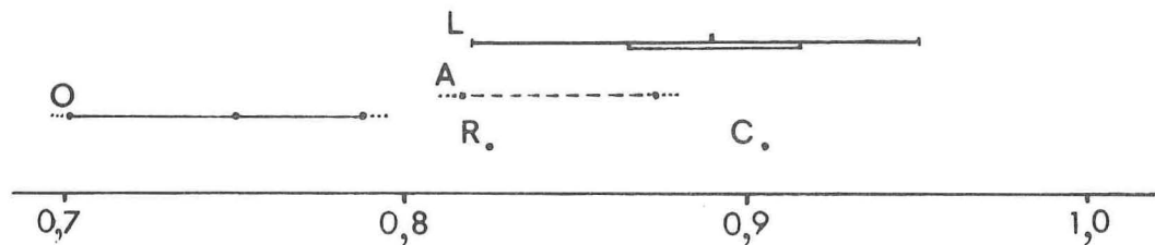
Figure 16. — Diagramme montrant la taille relative de différents Hyopsodus ; en abscisse : logarithme à base 10 du produit longueur \times largeur des M/1. L = intervalle de variation, moyenne et écart-type de cette dimension chez la plus ancienne population de H. loomisi du Wyoming (d'après Gingerich, 1976, a). A : deux points montrant la situation de H. wardi d'Angleterre, d'après les mesures de Hooker (1979). O : les trois points correspondant aux trois M/1 de H. orientalis d'après les mesures de Dashzeveg (1977). R. : la M/1 de Rians. C : la M/1 du Hyopsodus de Chine, d'après Zhai Renjie (1978).
