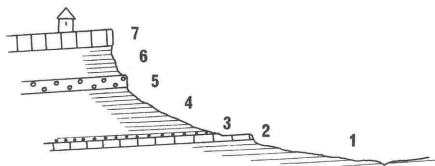
FIG. 3. — Coupe de l'Aquitanien de Caunelle d'après F. Roman.
