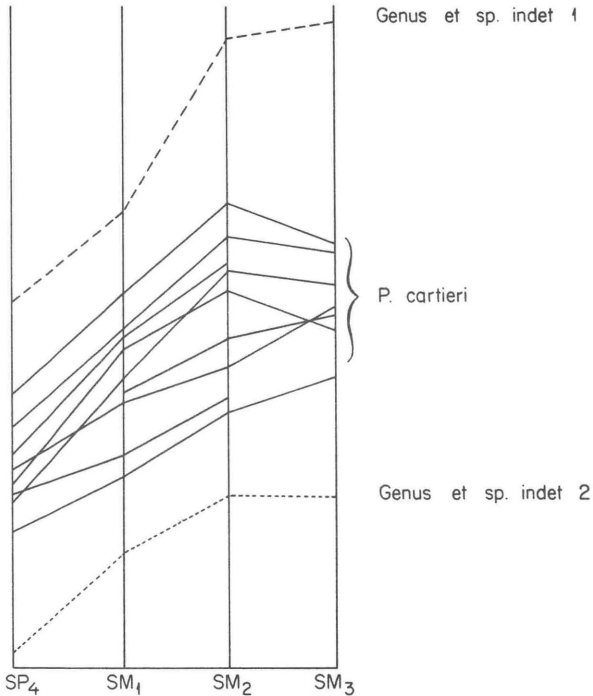
FIG. 4. — Profils arithmétiques correspondant aux surfaces des dents jugales inférieures de Protadelomys cartieri (Egerkingen \gamma , \alpha et Huppersand) et de Genus et species indet. 1 (Egerkingen \gamma ) et Genus et species indet. 2 (Egerkingen \alpha ).
