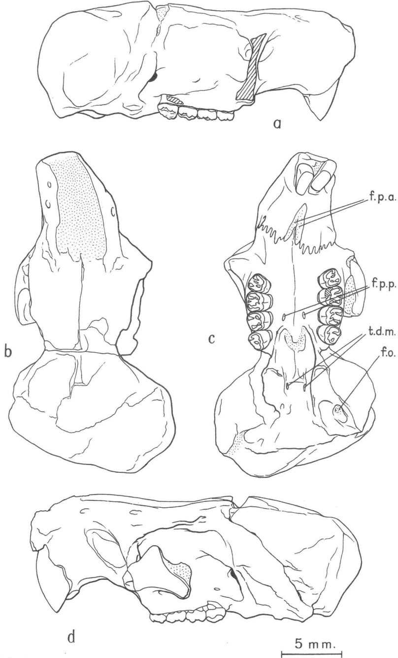
FIG. 2. — Protadelomys cartieri (STEHLIN et SCHAUB) : tête osseuse (Ek. 245, Musée de Bâle). Egerkingen γ.
