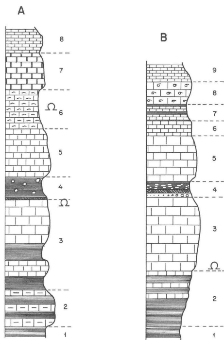
FIG. 3. — Coupes stratigraphiques détaillées de la base des Calcaires de Fons : A) à Robiac-Sud, B) à Robiac-Nord.
