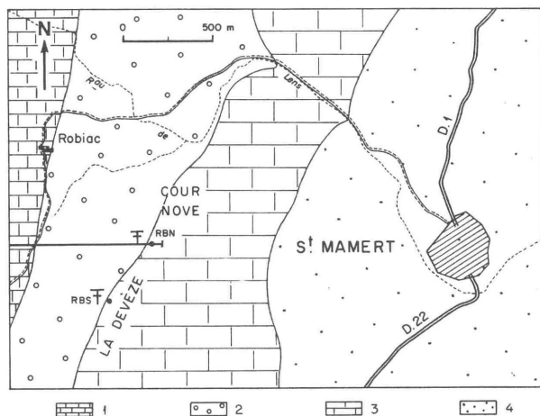
FIG. 1. — Esquisse géologique de la région de Saint-Mamert et situation des gisements de Robiac (RBN et RBS) : 1) Calcaires lacustres lutétiens, 2) Formation rouge de Robiac, 3) Calcaires de Fons, 4) Grès de Célas. (La coupe donnée Fig. 2 est indiquée)
