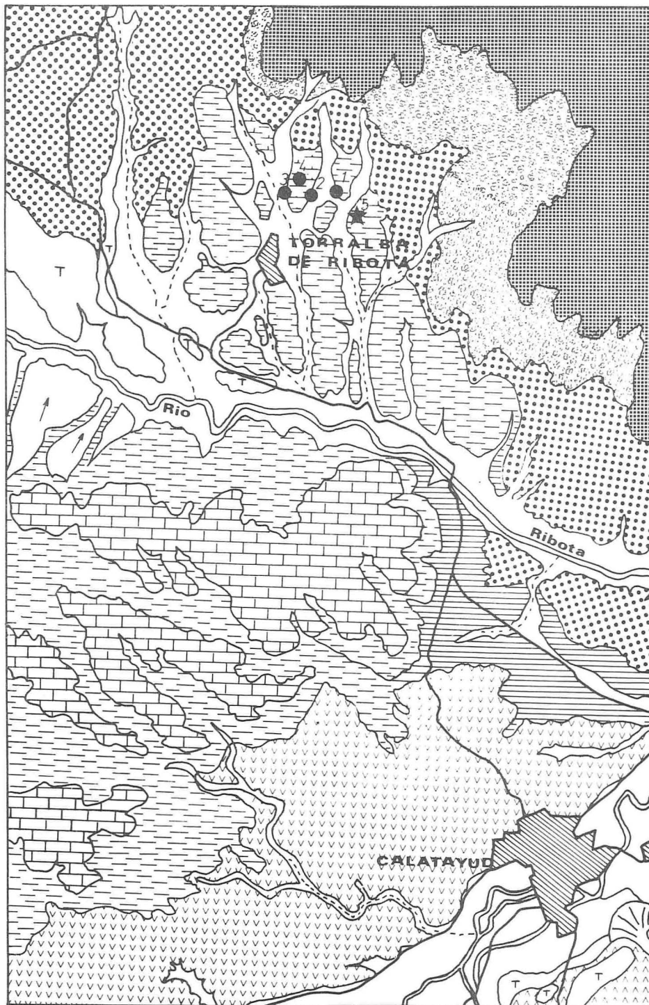
Fig. 2. — Géologie de la région de Calatayud — Torralba de Ribota.
