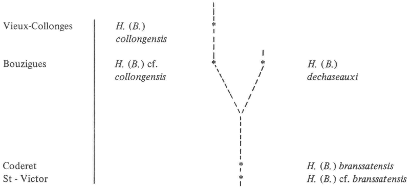
FIG. 18. — Schéma hypothétique de l'évolution des Brachipposideros tertiaires d'Europe.
