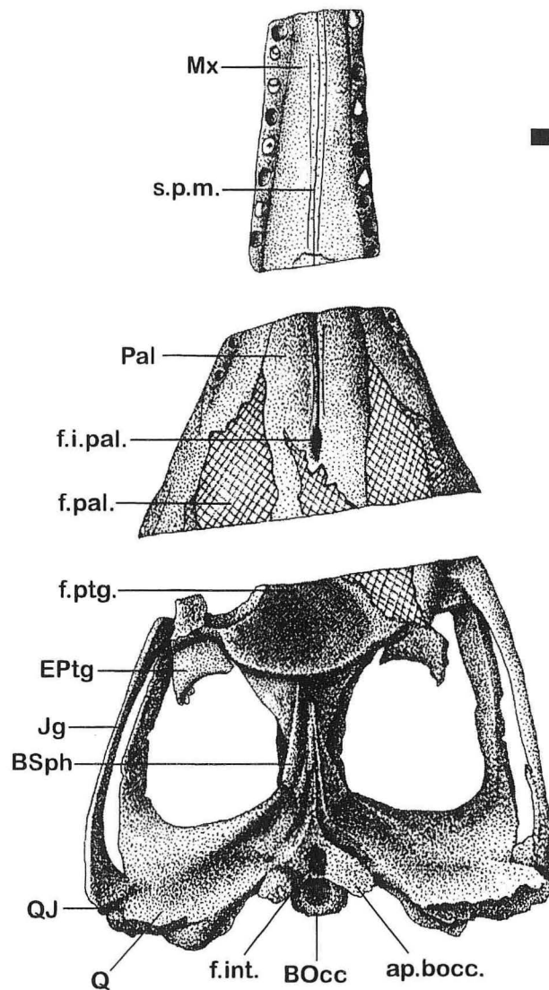
Figure 3b.— Steneosaurus pictaviensis n.sp. Holotype, crâne (LPP.M.35) face ventrale, zone à Coronatum, Migné-Auxances (Vienne, France). Barre d'échelle : 5 cm.
