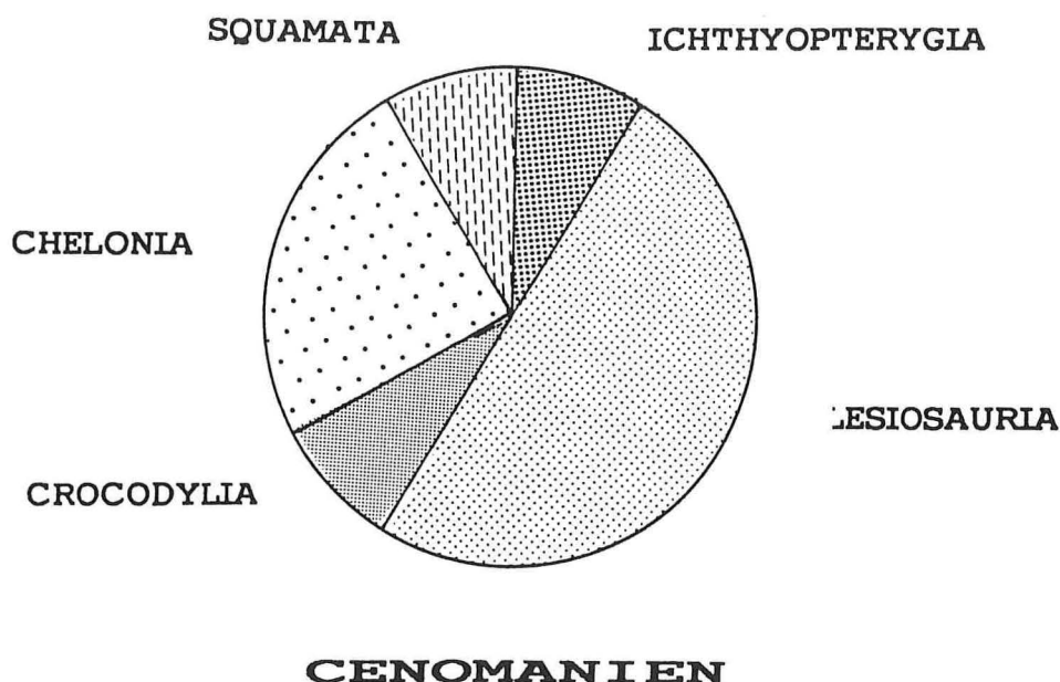
Figure 12.— Modèle de diversité des faunes de reptiles marins exprimé en pourcentage du nombre de genres au Cénomanien (Crétacé supérieur).
