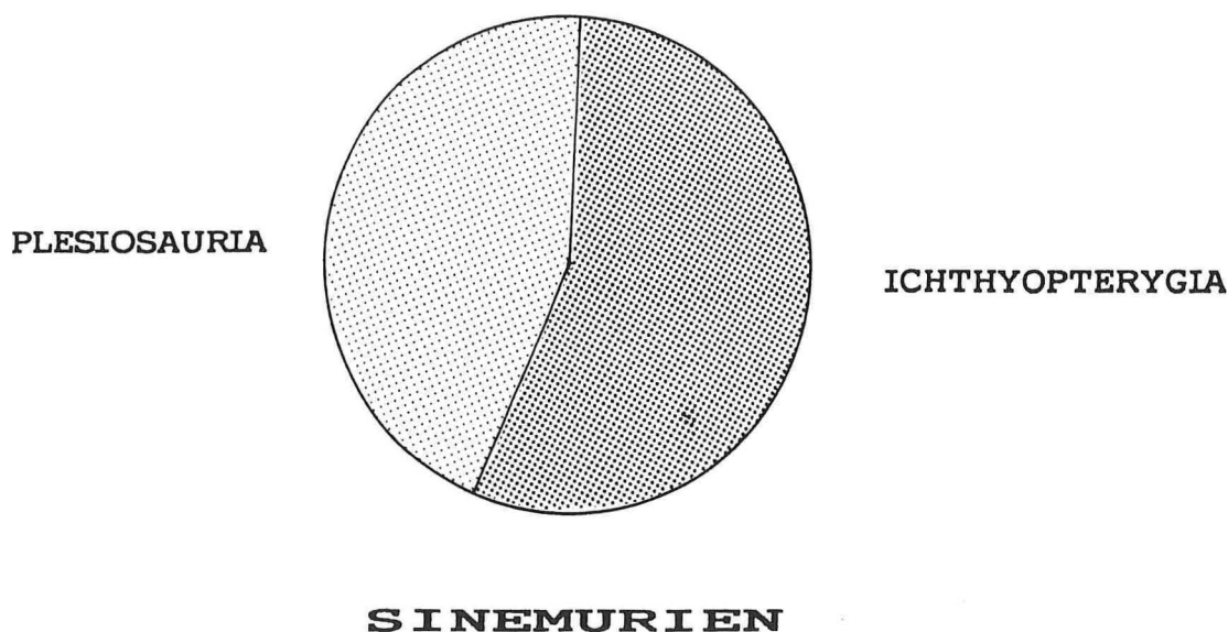
Figure 8.— Modèle de diversité des faunes de reptiles marins exprimé en pourcentage du nombre de genres au Sinémurien (Jurassique inférieur).
