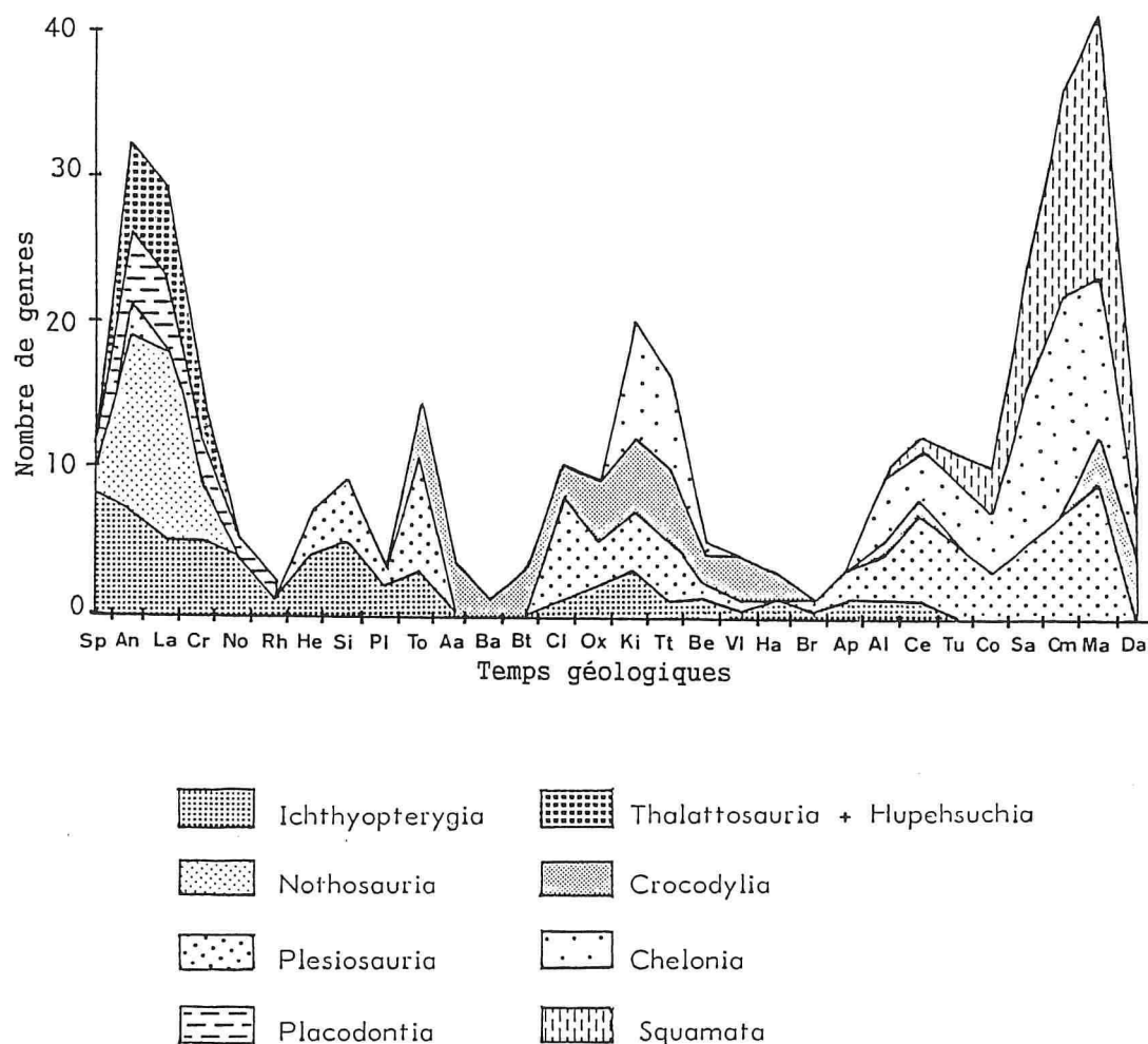
Figure 6.— Assemblages fauniques de reptiles marins mésozoïques du Trias inférieur (Spathien) au Paléogène (Danien).
