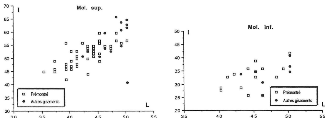
Figure 1.— Diagramme de dispersion établi à partir des Longueur (L), largeur (I), pour les molaires supérieures ( M^1 , M^2 , M^3 ) et inférieures ( M_1 , M_2 ) d' Eurodexis russelli nov sp. de Prémontré et d' Eurodexis cf. russelli de Cuis, St. Agnan, Grauves et Mancy.
