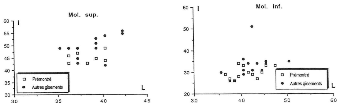
Figure 2.— Diagramme de dispersion établi à partir des Longueur (L), largeur (I) pour les molaires supérieures ( M^1 , M^2 , M^3 ) et inférieures du Diacodexis cf. varleti de Prémontré, Cuis, St. Agnan, Grauves et Mancy.
