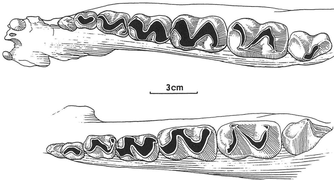
Figure 5.— Macrotherium macedonicum n. sp. Rangées dentaires inférieures DKO 234 (holotype), vue occlusale. Dytiko 3, Miocène supérieure; Université de Thessaloniki.
