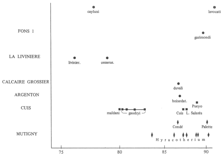
FIG. 6. — Evolution de l'indice de forme de la P⁴ (voir texte).
