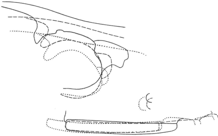
FIG. 14. — Superposition des profils faciaux de Pachynolophus lavocati n. sp., Pachynolophus livinierensis et Hyracotherium vulpiceps . Alignement sur le bord antérieur de l'orbite. (Mêmes figurés que Fig. 12) ( \times 1 ).
