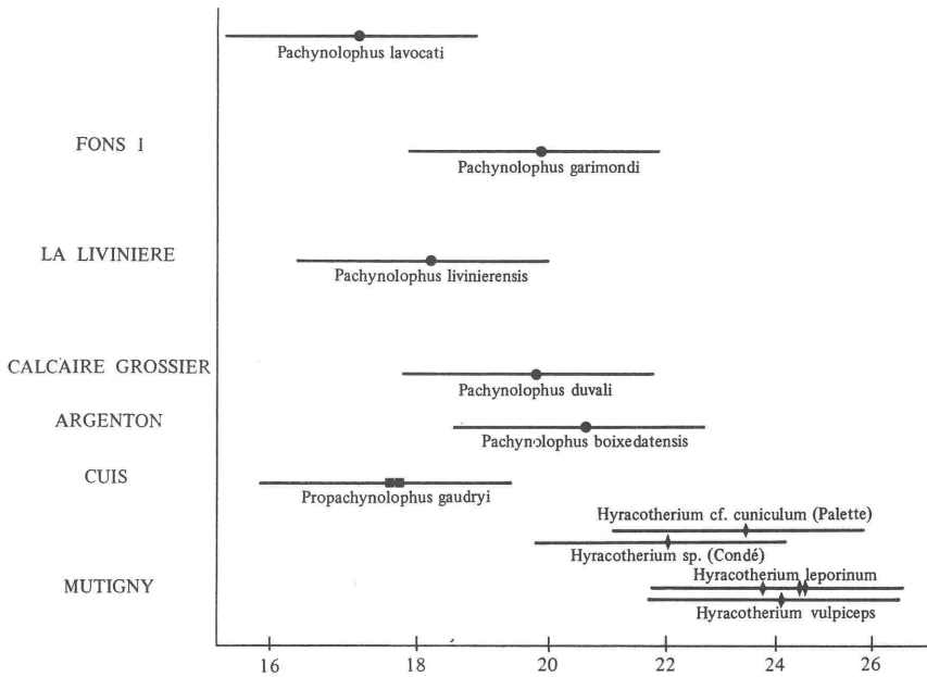
FIG. 4. — Evolution de la surface relative de P⁴ par rapport aux 3 M supérieures (en pourcentage).
