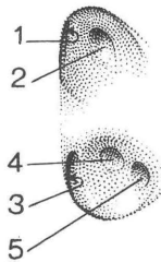
FIG. 11. — Conduit auditif interne droit.
