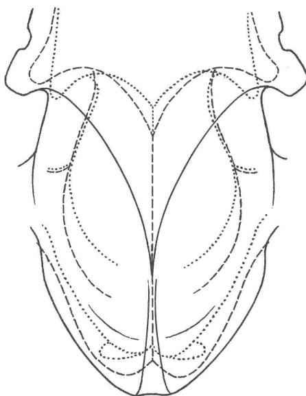
FIG. 12. — Superposition en plan des crânes de Pachynolophus lavocati n.sp. (—), Pachynolophus livinierensis (---) et Hyracotherium vulpiceps (.....). Alignement sur la constriction post-orbitaire ( \times 1 ).
