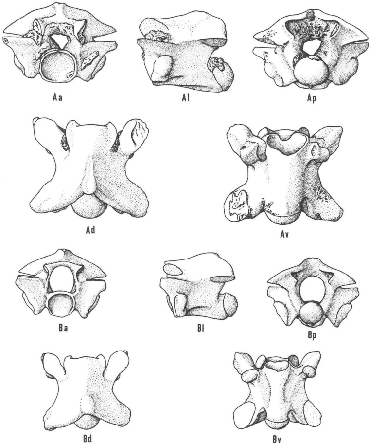
FIG. 1. — Eoanilius europae nov. gen., n. sp., Malpérié; x 10.
