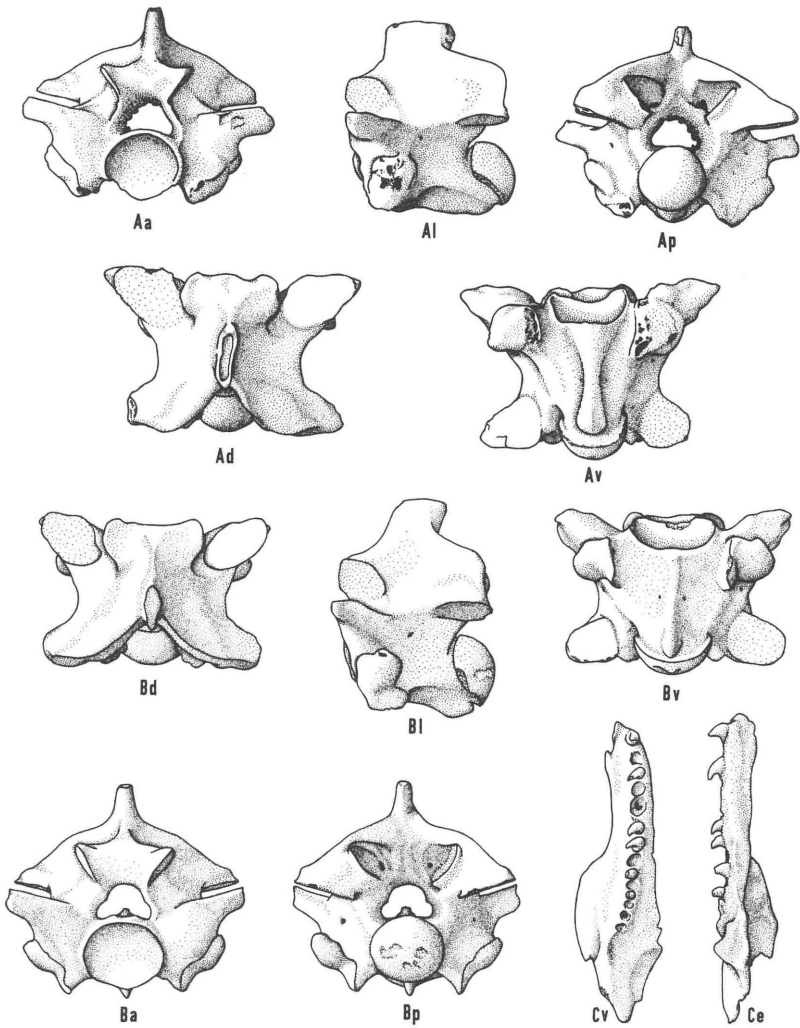
FIG. 3. — Palaeopython filholi ; x 2.
