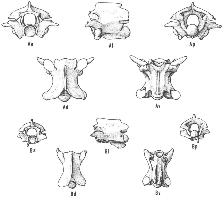
FIG. 7. — Coluber cadurci n. sp., Mas-de-Got locus A; x 5.
