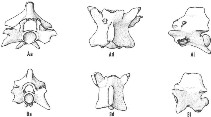
FIG. 5. — Platyspondylia lepta nov. gen., n. sp., Pech-du-Fraysse; x 7. A : vertèbre caudale antérieure (PFR 6353; Muséum, Paris); B : vertèbre caudale postérieure (PFR 6354; Muséum, Paris). Faces antérieure (a), dorsale (d) et latérale (l).
