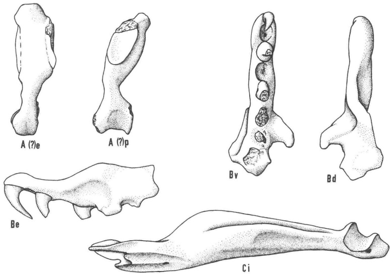
FIG. 6. — Platyspondylia lepta nov. gen., n. sp., Pech-du-Fraysse; x 10. A : quadratum, (?) gauche (PFR 6355; Muséum, Paris); B : palatin gauche (PFR 6356; Muséum, Paris); C : articulaire s.l. (PFR 6357; Muséum, Paris). Faces ventrale (v), dorsale (d), externe (e), postérieure (p) et interne (i).
