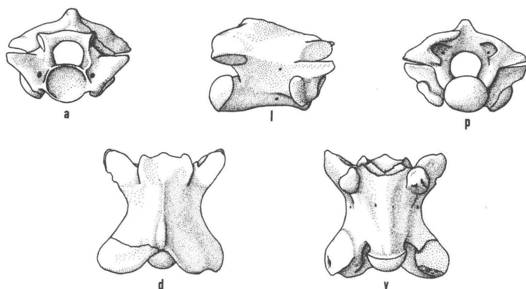
FIG. 8. — Dunnophis cadurcensis n. sp., Malpérié; x 8.
