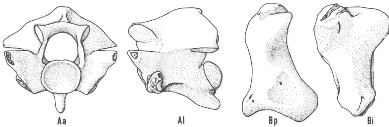
FIG. 2. — Eoanilius europae nov. gen., n. sp., Malpérié; x 10. A : vertèbre dorsale antérieure (MAL 552, Univ. Montpellier); B : quadratum droit (MAL 553, Univ. Montpellier). Faces antérieure (a), latérale (l), postérieure (p) et interne (i).
