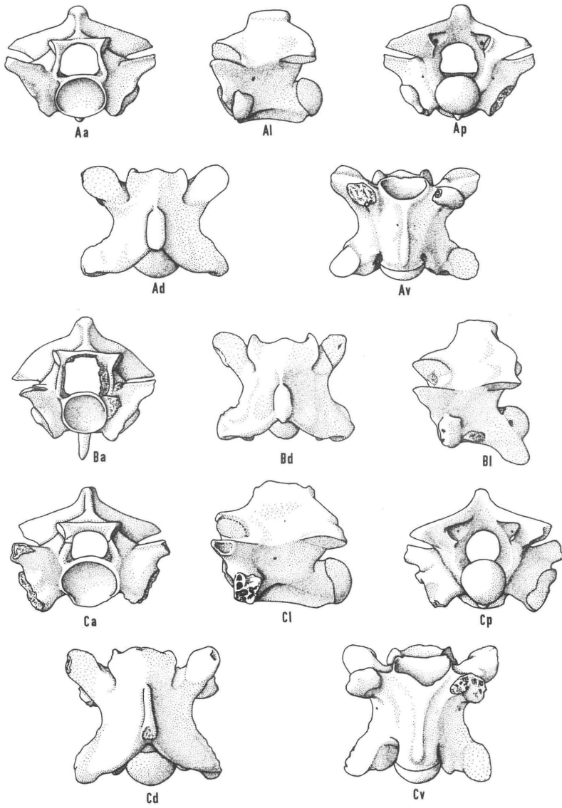
FIG. 4. — Platyspondylia lepta nov. gen., n. sp., Pech-du-Frayse; x 7. A : vertèbre dorsale moyenne, type (PFR 6350, Muséum, Paris); B : vertèbre dorsale antérieure (PFR 6351; Muséum, Paris); C : vertèbre dorsale postérieure (PFR 6352; Muséum, Paris). Faces antérieure (a), latérale (l), postérieure (p), dorsale (d) et ventrale (v).
