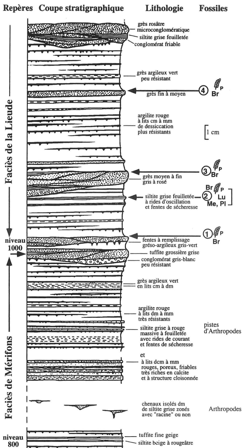
Figure 4.— Coupe lithologique de la partie de la Formation du Salagou contenant les niveaux à traces de vertébrés tétrapodes de la Lieude; 2-3 = site B ou RNV et 3 = site A à Brontopus giganteus ; 2 = niveau à Br = Brontopus , Lu = Lunaepes , Me = Merifontichnus , Pl. = Planipes .
