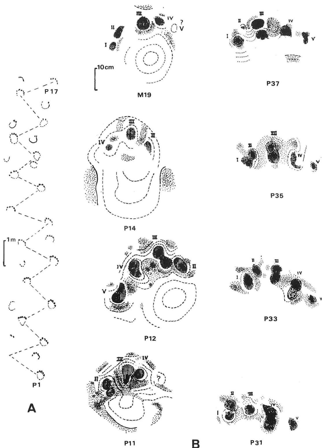
Figure 23.— A : piste 13 Brontopus circagiganteus nov. ichnosp., de P1 à P17. B : Quelques mains (= M) et pieds (= P) Brontopus circagiganteus nov. ichnosp. de la piste 13; le pointillé représente le sédiment refoulé et les hachures, les griffes; holotype : pied = P33.13 et main = M19.13.
