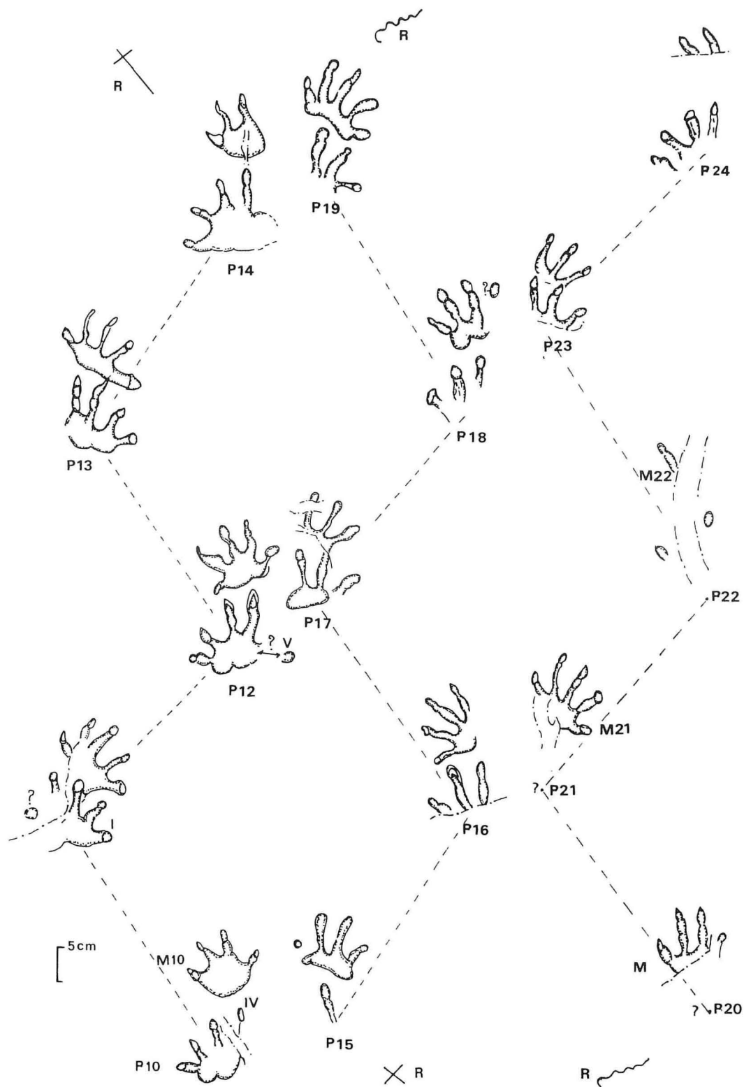
Figure 14.— Piste n° 2 Merifontichnus thalerius nov. ichnogen. et nov. ichnosp., de P10 à P24; P13 = pied = holotype, R = repère pour aligner la piste 2 de P10 à P24.
