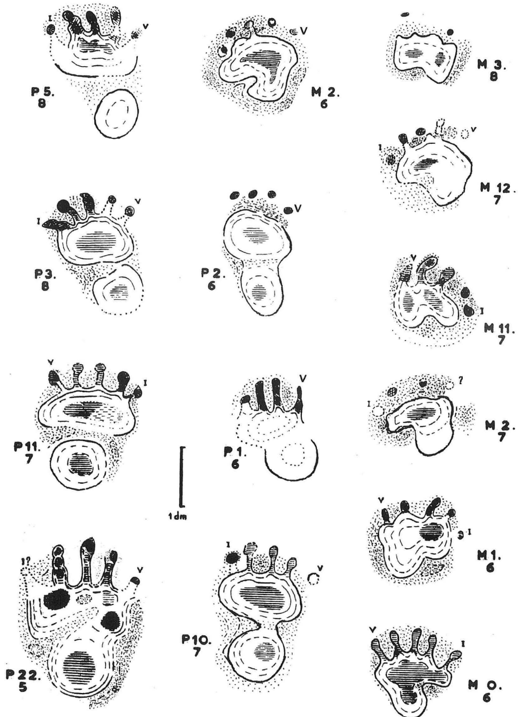
Figure 17.— Quelques mains (= M) et pieds (= P) Planipes brachydactylus nov. ichnosp.; holotype : main = M2 de la piste 6 (M2.6) et pied = P11 de la piste 7 (P11.7).
