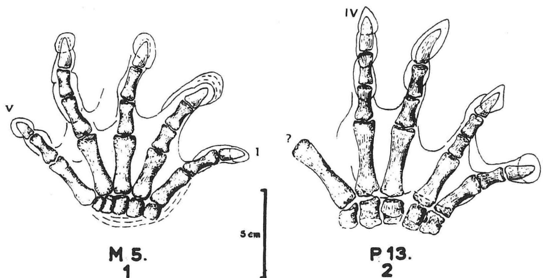
Figure 16.— Essai de reconstruction squelettique de l'acropode, du métapode et d'une partie du basipode de Merifontichnus thalerius nov. ichnogen. et nov. ichnosp.
