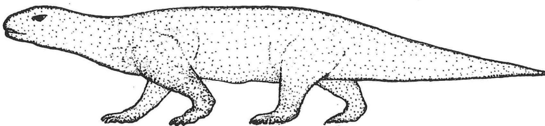
Figure 25.— Silhouette possible de l'ichnopoïète de Brontopus circagiganteus nov. ichnosp., piste 13, attribué à un Therapsida ou à un Caseomorpha (x 1/40).
